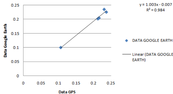
Gambar 2. GrafikValidasiLuasanSawah
